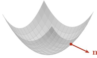
Şekil 1.3: z = x^2 + y^2 paraboloidi ve bir noktasındaki normal vektörü \mathbf{n} = (2a, 2b, -1) . z bileşeni -1 olduğu için vektör aşağıya, yüzeyin dışına bakar.
