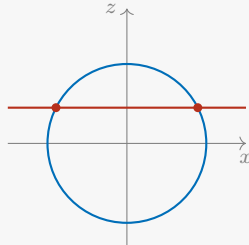
c_1^2 > c_2^2 : çember
