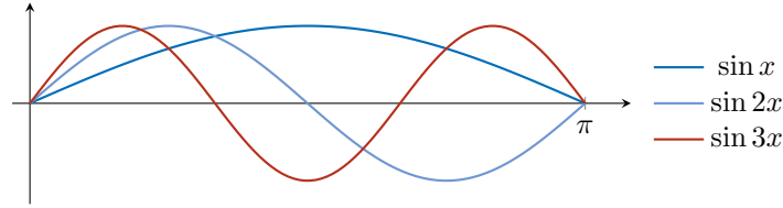
Şekil 1.2: X'' - \lambda X = 0 , X(0) = X(\pi) = 0 sınır değer probleminin sıfır olmayan çözümleri: \sin nx , n = 1, 2, 3 .
