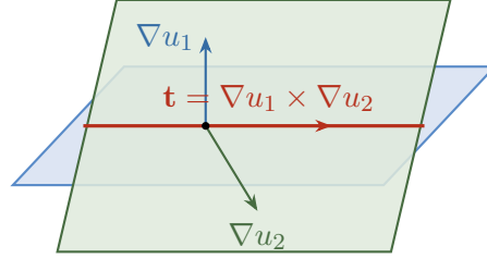
Şekil 1.5: İki düzlemin kesişimi bir doğrudur. Kesişim doğrusunun doğrultusu iki normale de dik, yani \nabla u_1 \times \nabla u_2 yönündedir.
