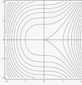
Şekil 1.1: Farklı c değerleri için \frac{y^2}{2} - \frac{x^3}{3} = c denkleminin seviye eğrileri.
